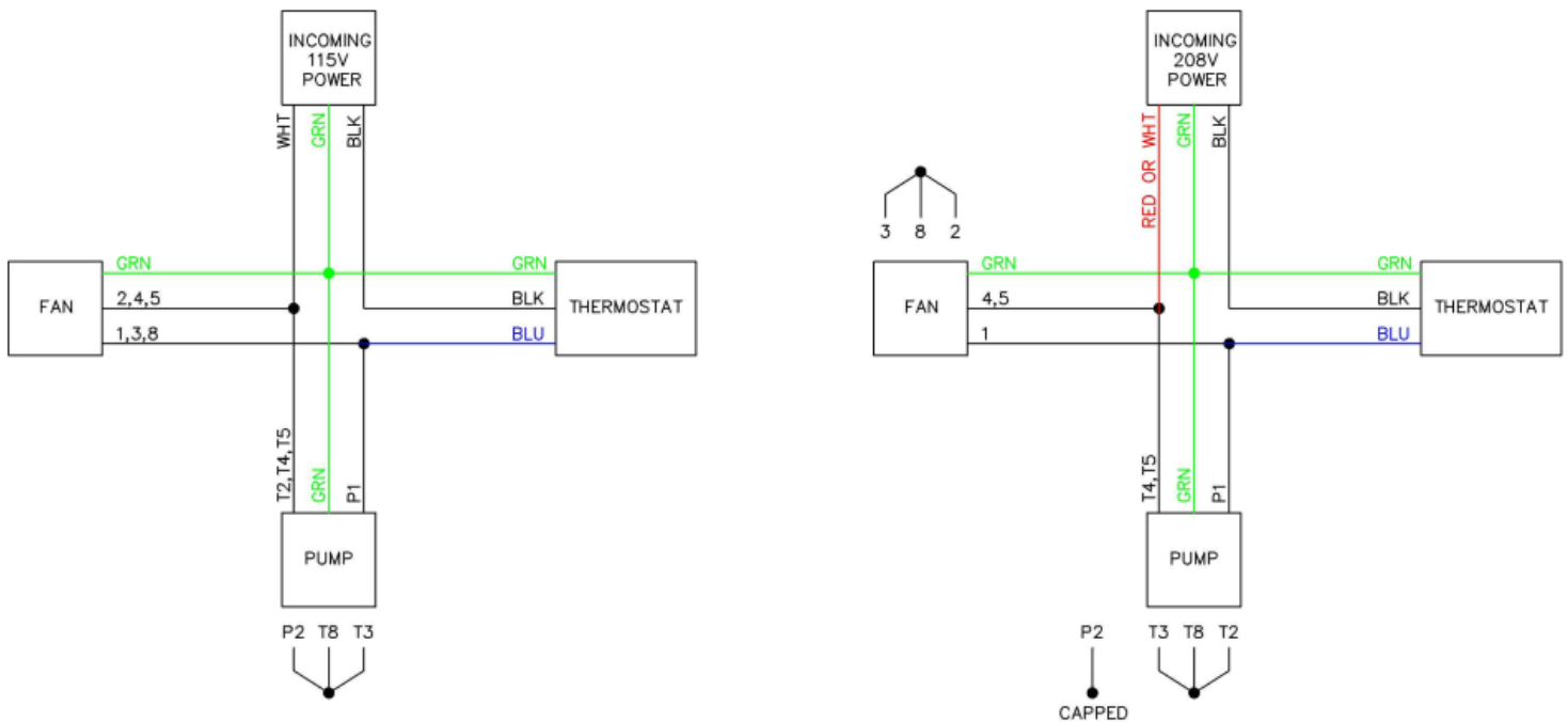
Fig. 13: Wiring diagram.
